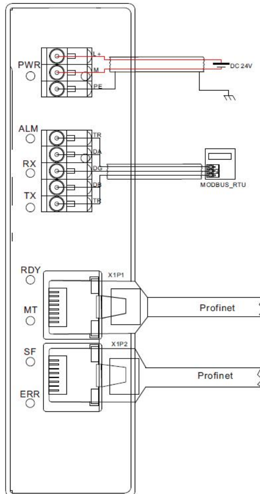
图 1: 接线图
