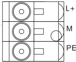
图 2: 电源接口
